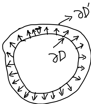
图 2.3: 流体中某个区域随着流体流动经过 dt 时间之后的体积改变。
