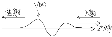
Figure 11.3: 自由粒子从势 V(x) 的右边入射。
