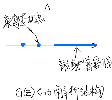
Figure 10.5: G(z) 的解析结构, 束缚态对应实轴上的极点。
