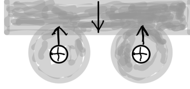
Figure 5.7: 铁磁体通过共享的传导电子而自旋平行
