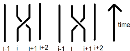
Figure 8.5: 左图是 \sigma_i ，右图是 \sigma_i^{-1} 。(图片来自于网络)
