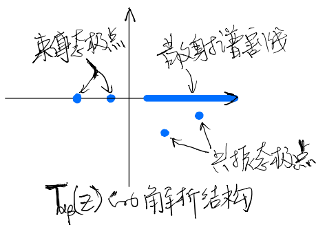
Figure 10.6: T_{\alpha\beta}(z) 的解析结构。
